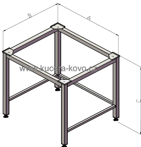
typ P-T
