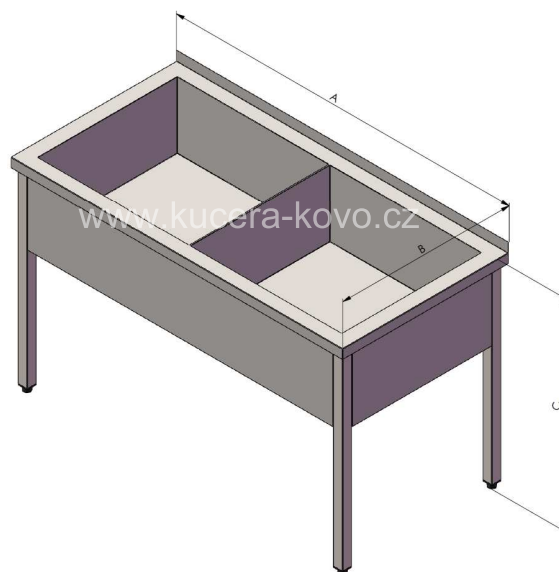
Dvoudřez MS-ST
