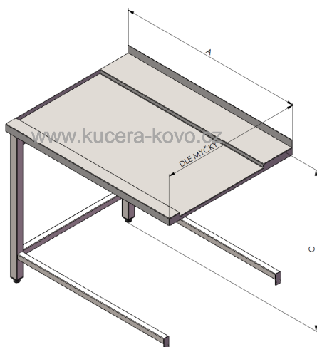
VSM-ZL (levý)
