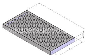
odkapní vanička
